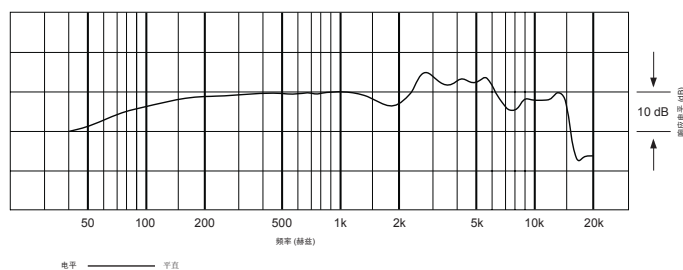
频率特性
