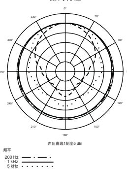
指向特性
